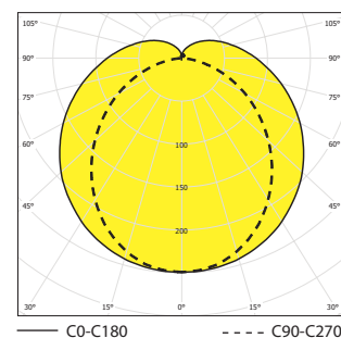
AQUARI-LED-OP-4K, IP68
