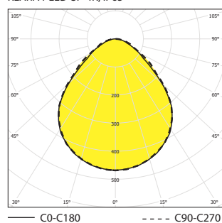
KLARA4-LED-SP-4K, IP65
